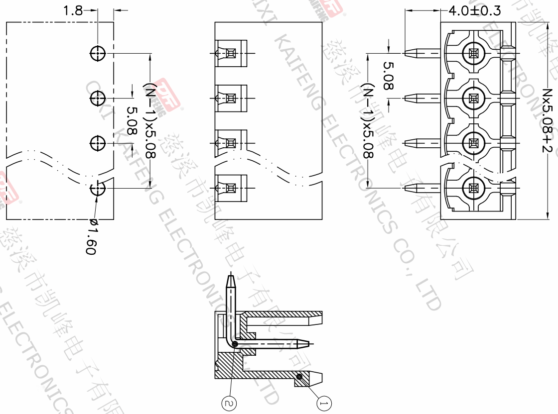
P.C.B.LAYOUT
