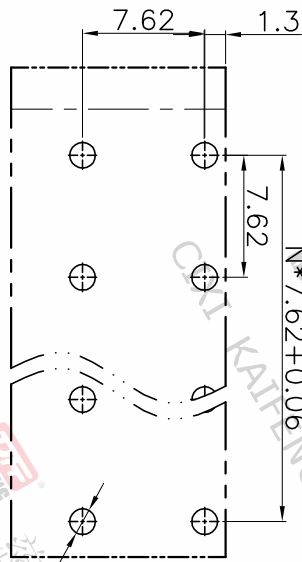
P.C.B.LAYOUT
