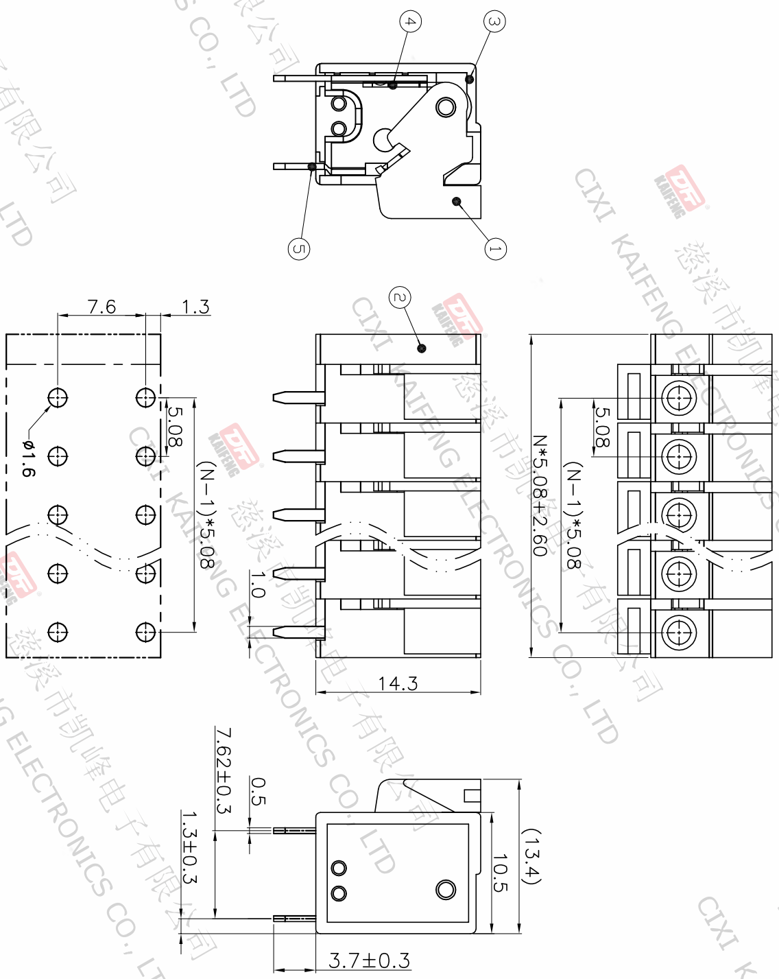
P.C.B.LAYOUT
