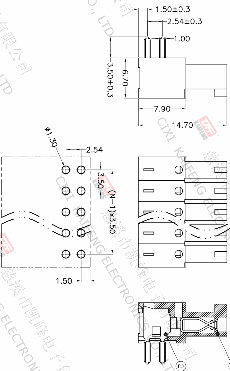
P.C.B.LAYOUT
